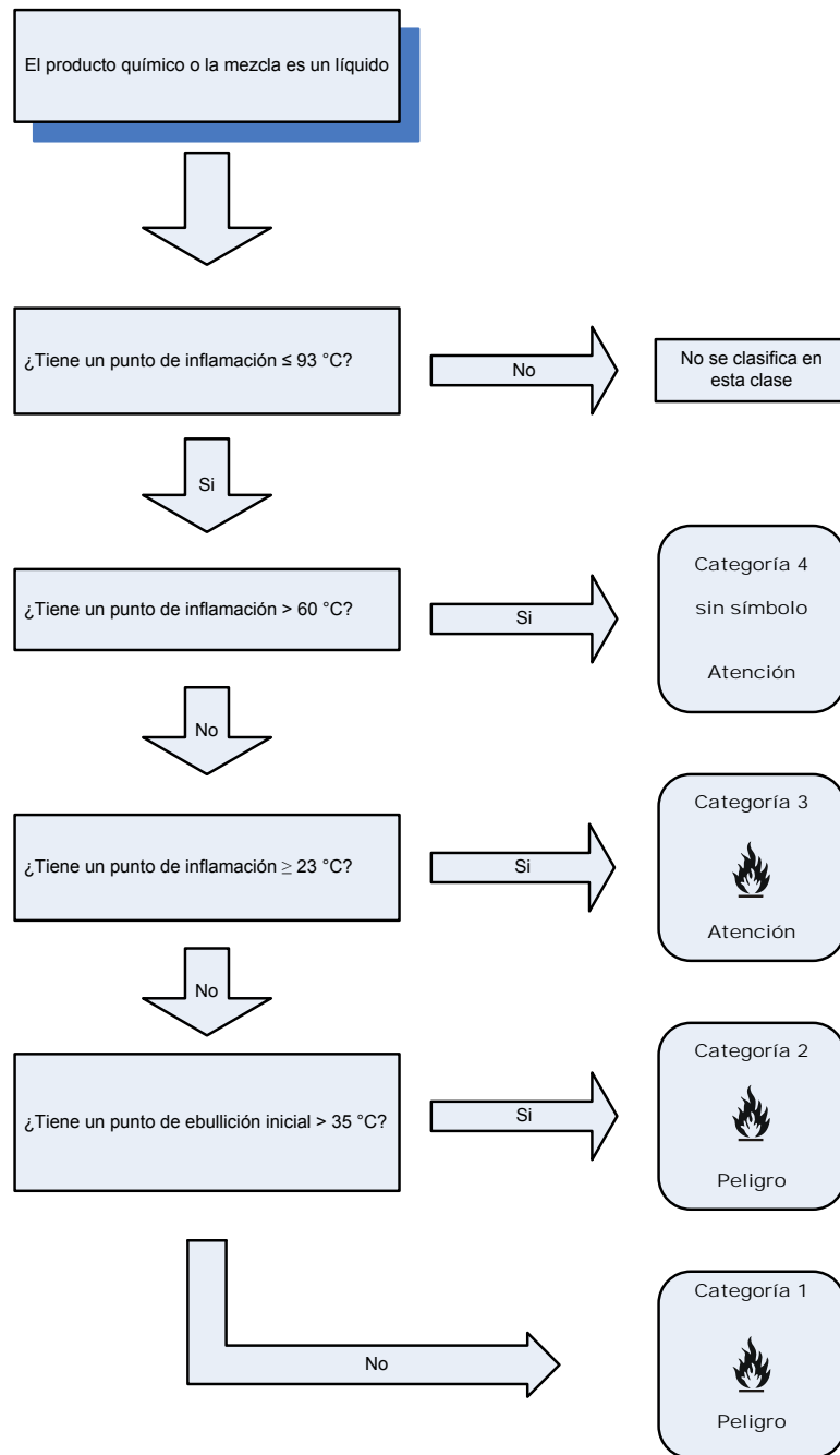
FIGURA 7. Procedimiento de decisión para líquidos inflamables.
