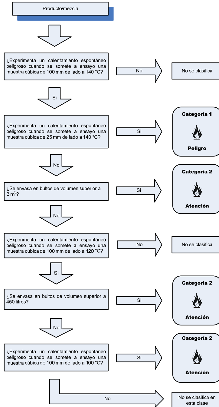
FIGURA 12. Procedimiento de decisión para sustancias y mezclas que experimentan calentamiento espontáneo.
