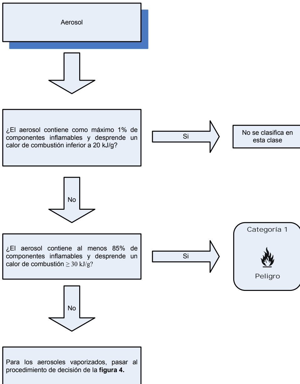
FIGURA 3. Procedimiento de decisión para aerosoles inflamables.
