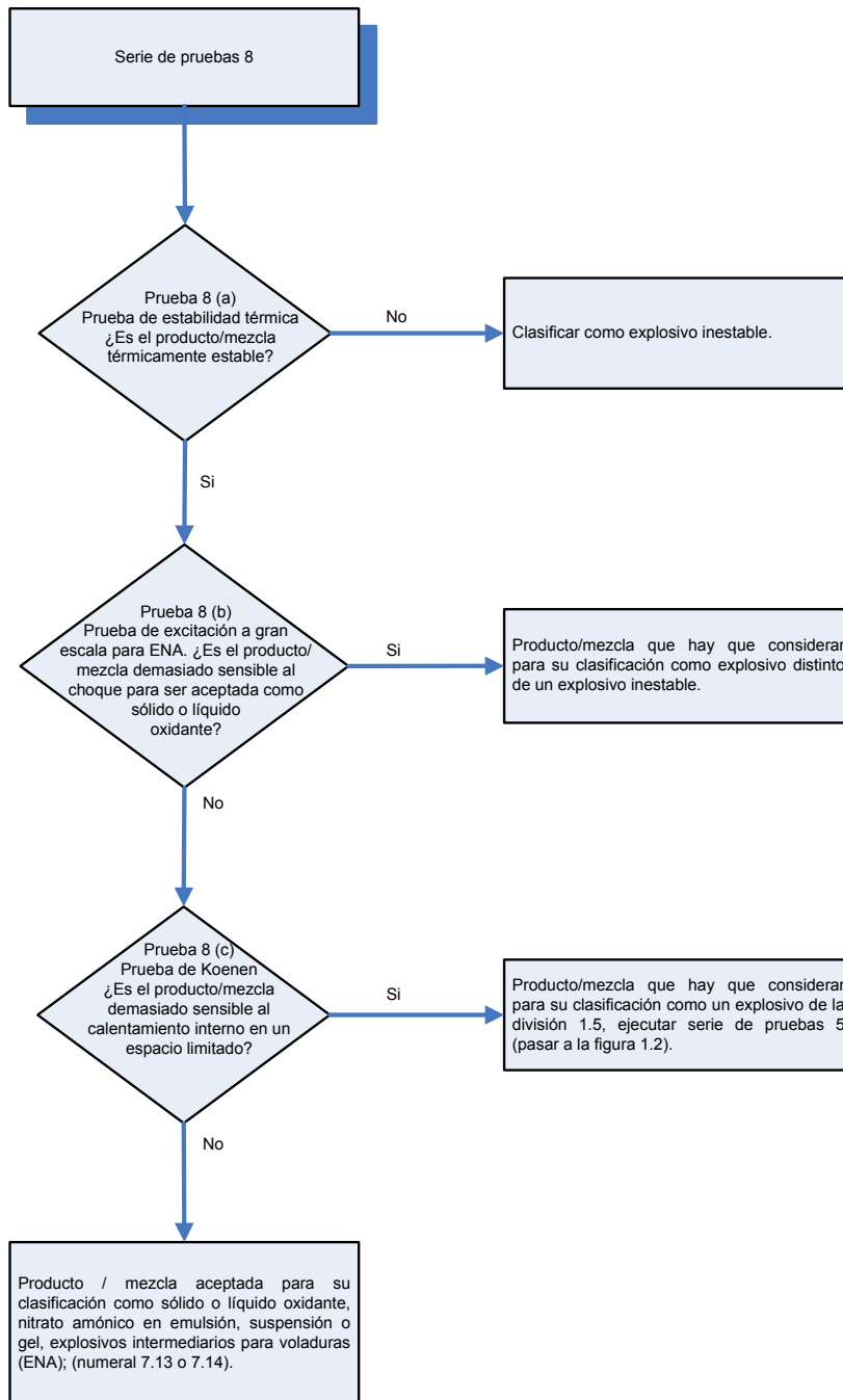
FIGURA 1.2. Procedimiento para la clasificación de Nitrato de Amonio en suspensión emulsión o gel.
