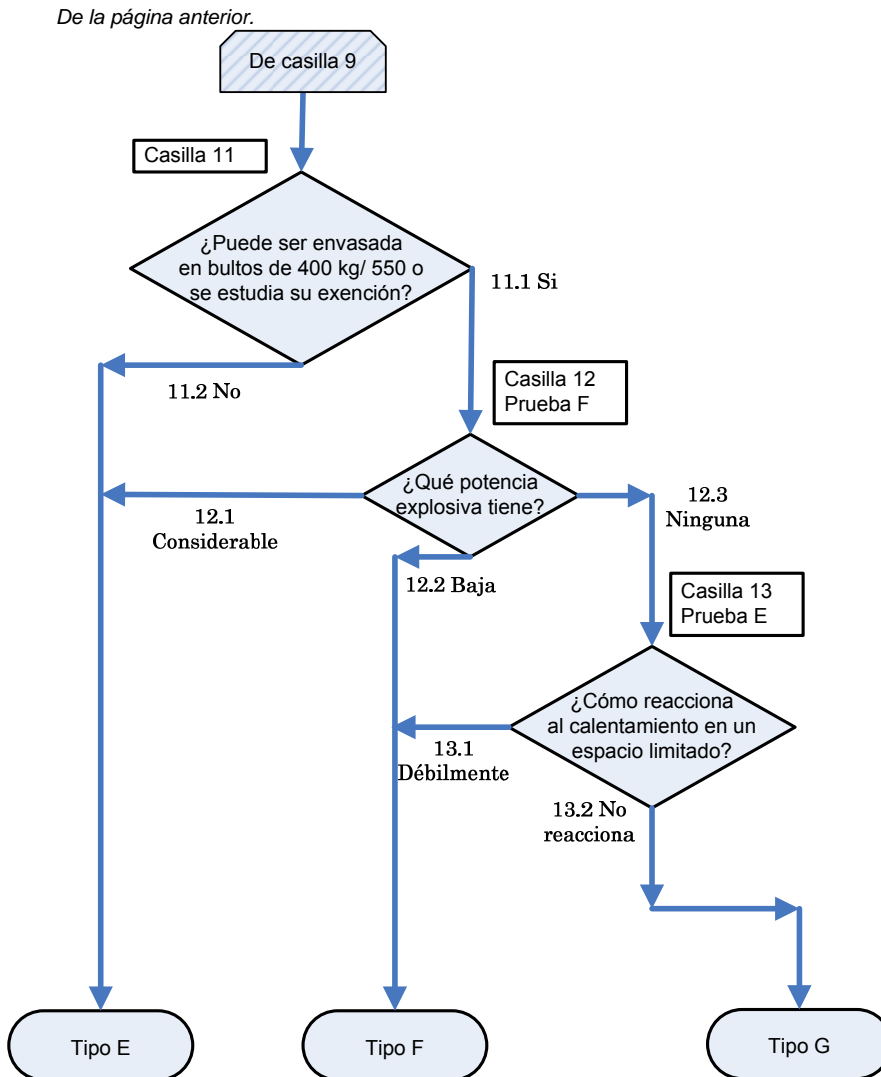
FIGURA 9. Procedimiento de decisión para sustancias y mezclas que reaccionar espontáneamente.
