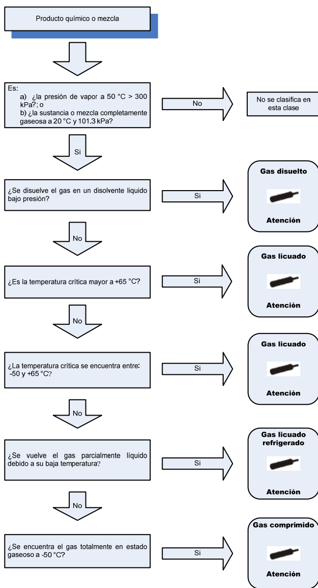
FIGURA 6. Procedimiento de decisión para gases a presión.
