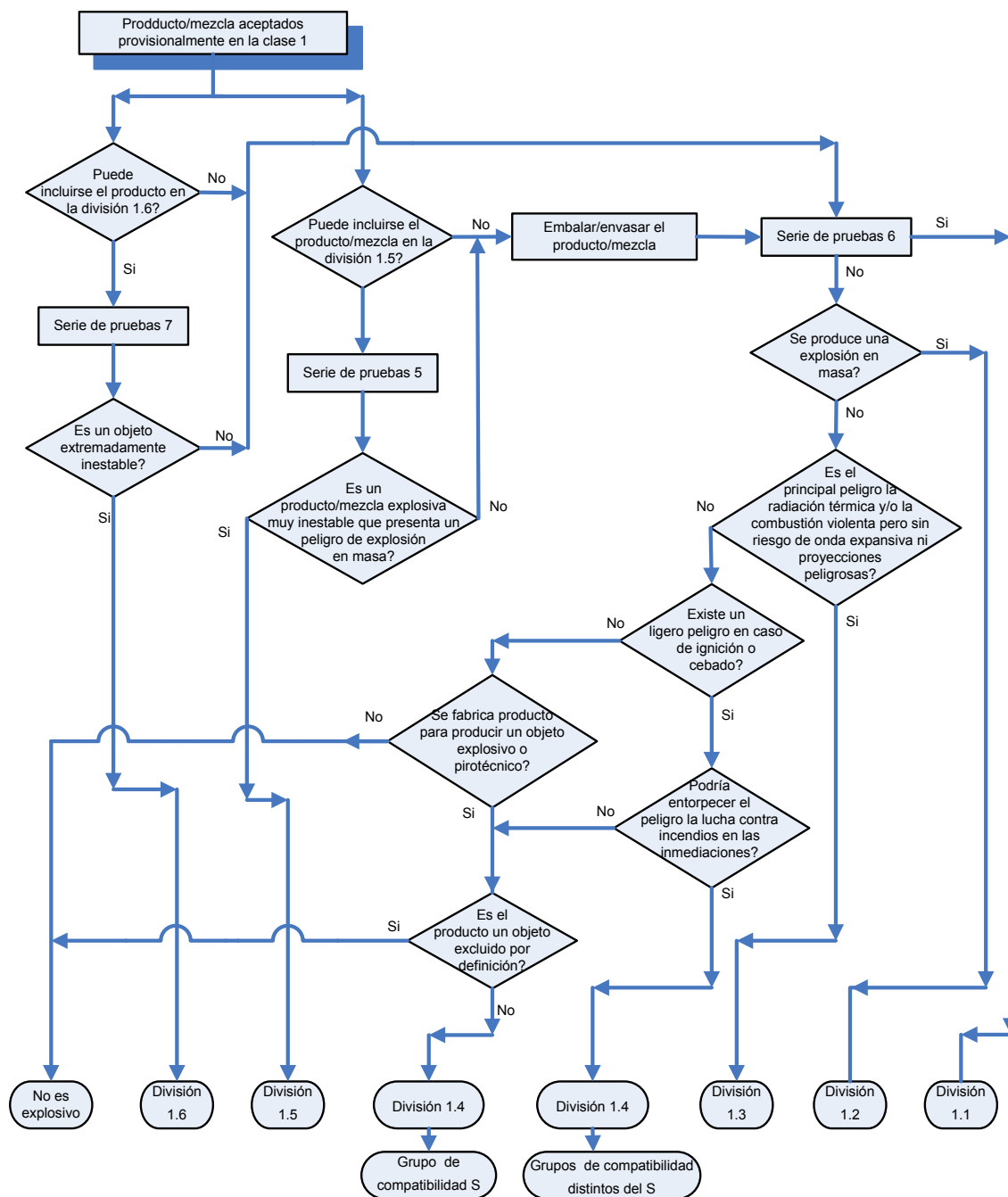
FIGURA 1.1. Procedimiento de asignación a una división de la clase de explosivos (Clase 1 para el transporte)
