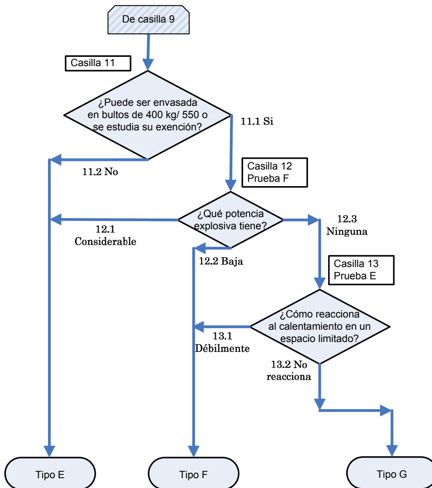
FIGURA 16. Procedimiento de decisión para peróxidos orgánicos.
