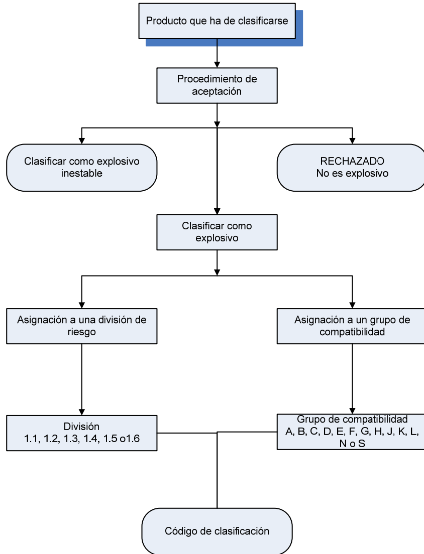
FIGURA 1: Esquema general del procedimiento de decisión para clasificar una sustancia, mezcla o artefacto explosivo en la clase de explosivos (Clase 1 para el transporte).
