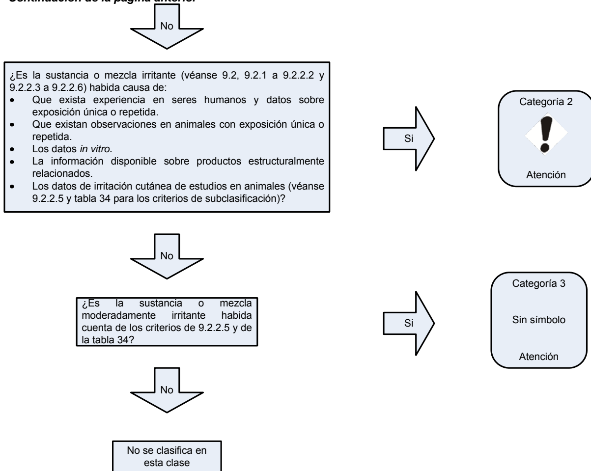
FIGURA 21. Procedimiento de decisión para productos químicos corrosivos o irritantes a la piel
