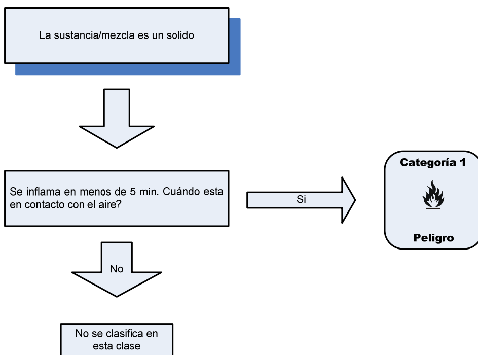
FIGURA 11. Procedimiento de decisión para sólidos pirofóricos.
