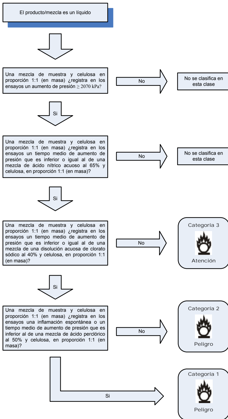
FIGURA 14. Procedimiento de decisión para líquidos oxidantes.
