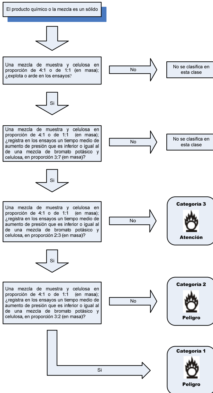
FIGURA 15. Procedimiento de decisión para sólidos oxidantes.
