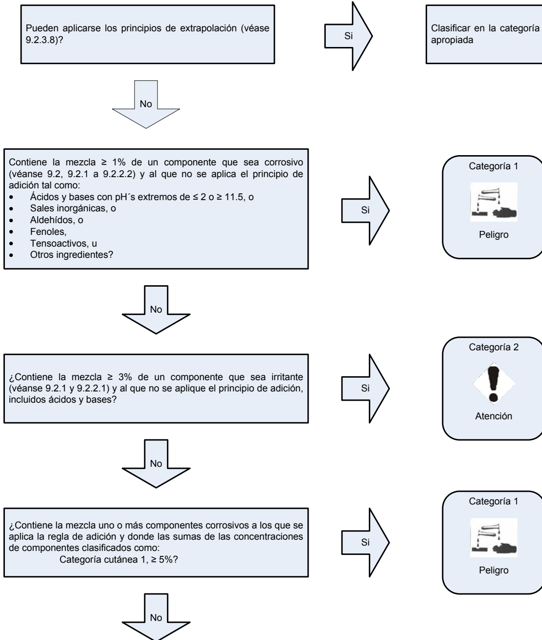
FIGURA 22. Procedimiento de decisión para productos químicos corrosivos o irritantes a la piel. Clasificación de mezclas en base a la información de los componentes.
