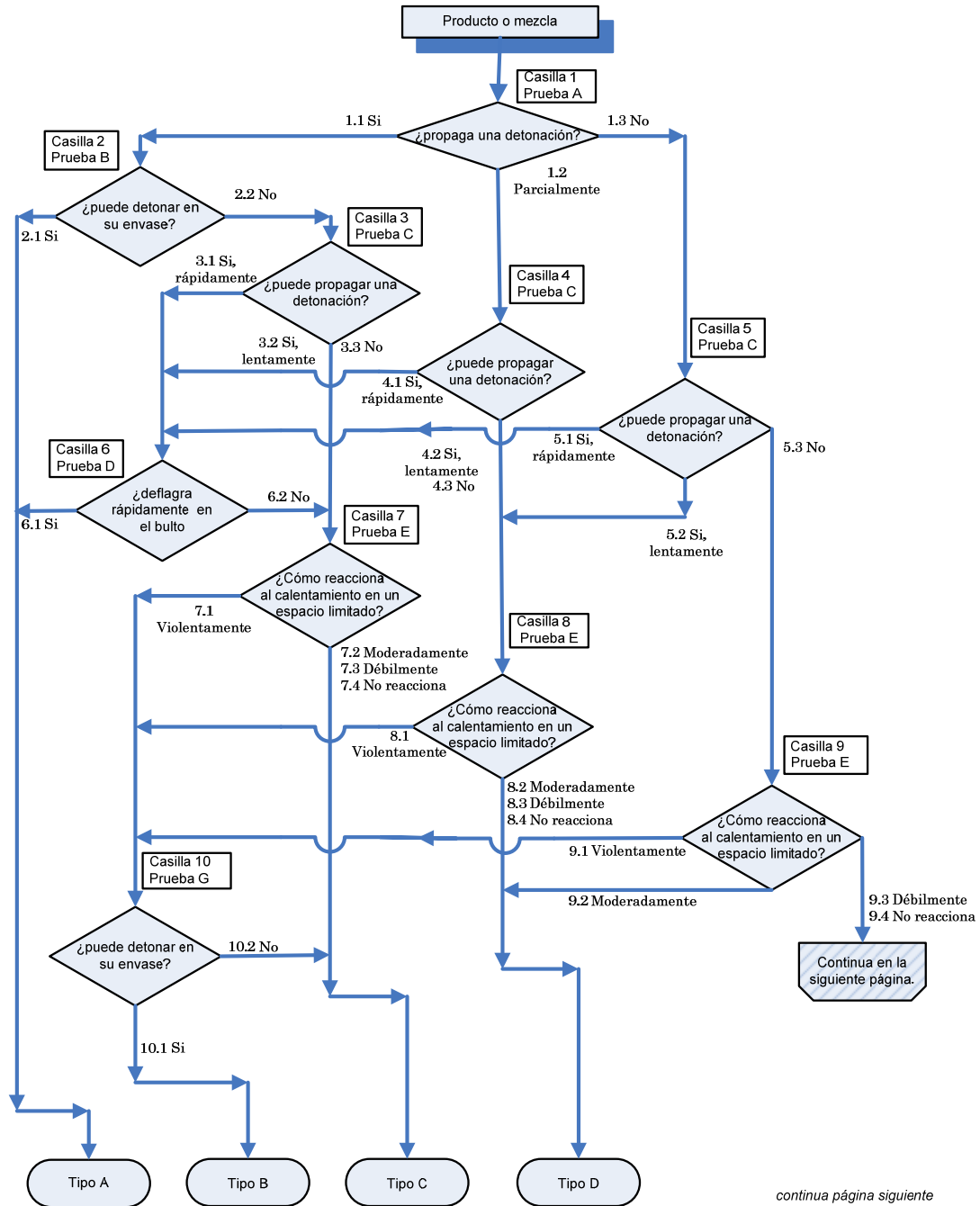
FIGURA 16. Procedimiento de decisión para peróxidos orgánicos.
