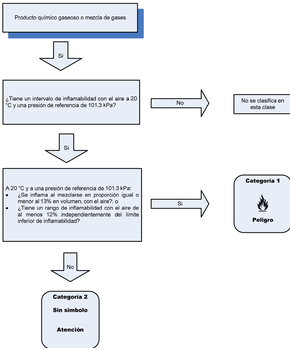
FIGURA 2. Procedimiento de decisión para la clasificación de gases inflamables.
