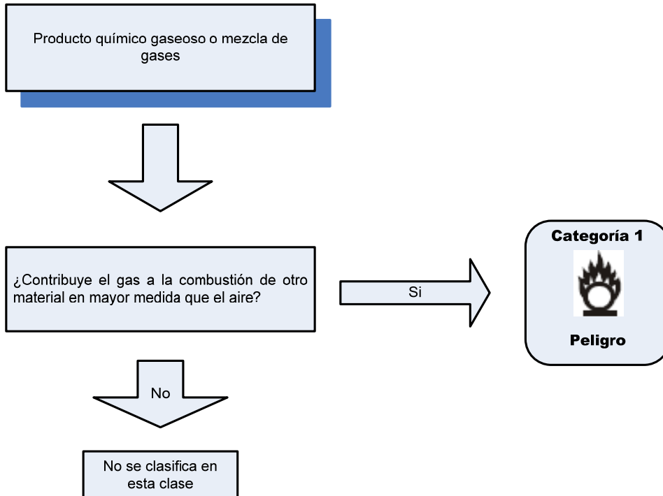
FIGURA 5. Procedimiento de decisión para gases oxidantes.
