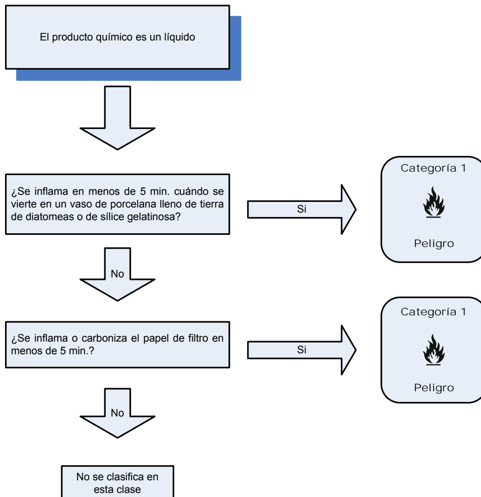
FIGURA 10. Procedimiento de decisión para líquidos pirofóricos.
